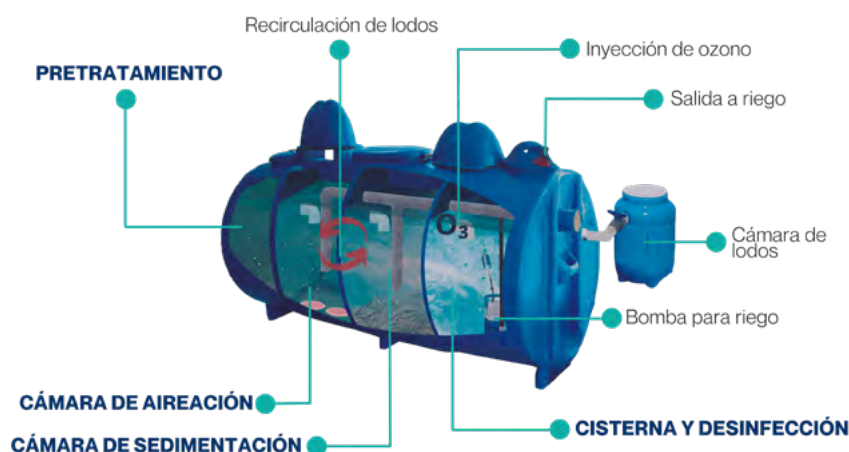
ESQUEMA BIOGEST PLUS STAR
