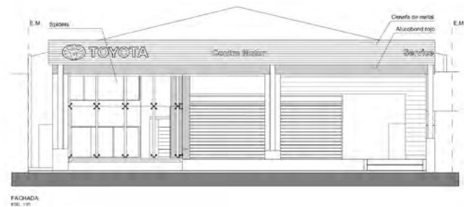
Fachada
