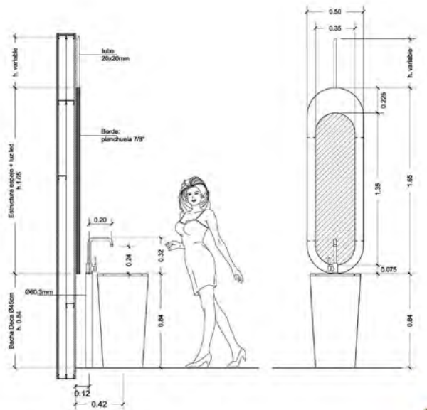
DETALLE DE BACHAS Y ESPEJOS BAÑO
