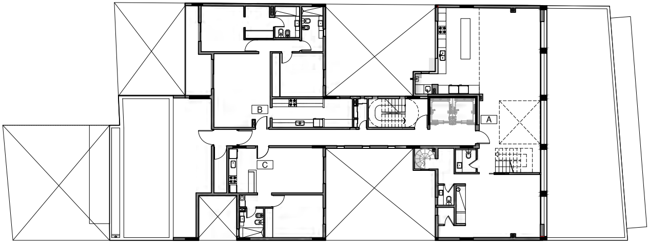
PLANTA NIVEL 12° ESC 1:200
