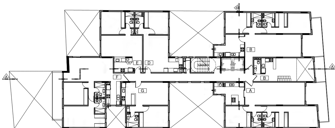
PLANTA TIPO NIVELES 1° A 8° ESC 1:200
