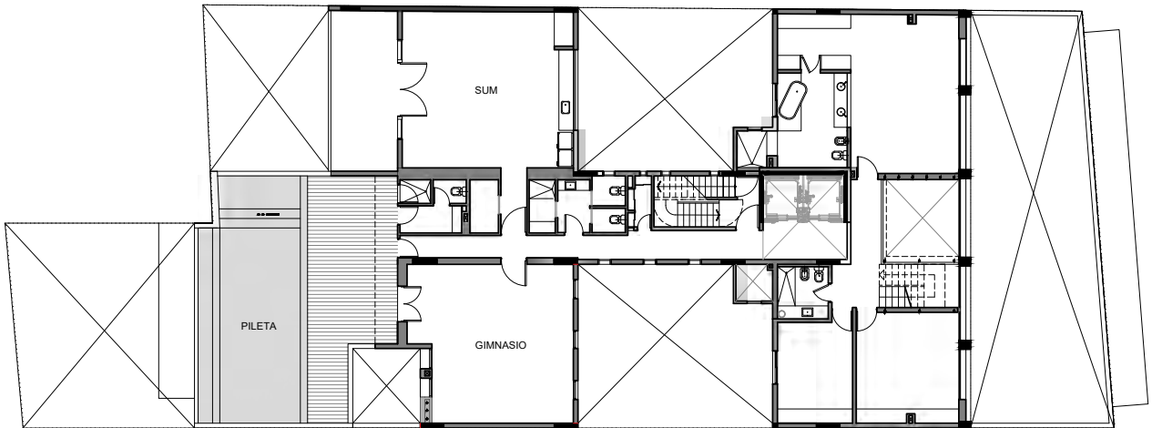
PLANTA NIVEL 13° ESC 1:200
