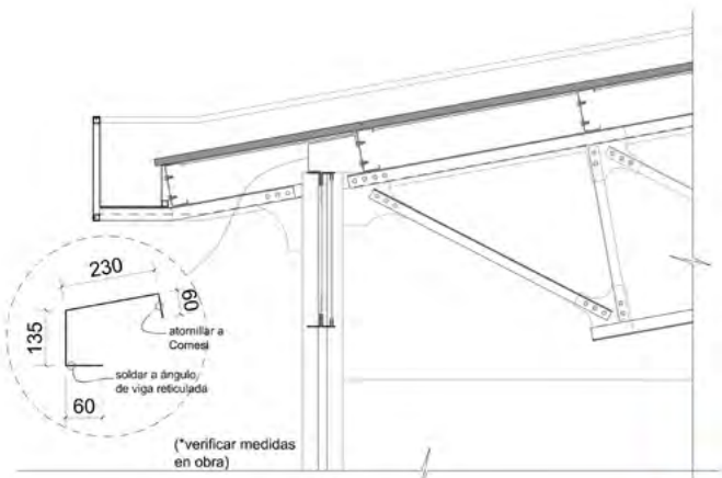
DETALLE CERRAMIENTO ALERO - FACHADA
