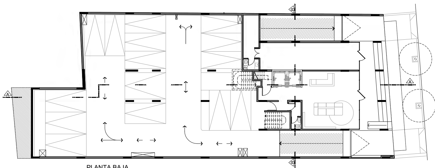
PLANTA BAJA ESC 1:200
