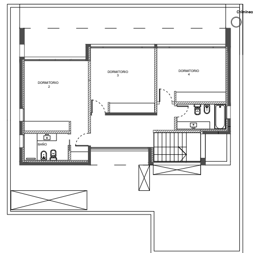
PLANTA ALTA
